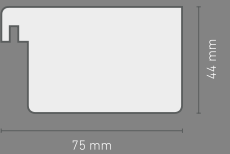
Aufbau Blendrahmen Blind frame construction
