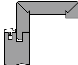
ZARGE MIT RUNDKANTE, 60 MM BEKLEIDUNG FRAME WITH ROUNDED EDGE, 60 MM CASING
