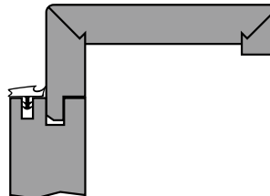
ZARGE MIT RUNDKANTE, 100 MM BEKLEIDUNG FRAME WITH ROUNDED EDGE, 100 MM CASING
